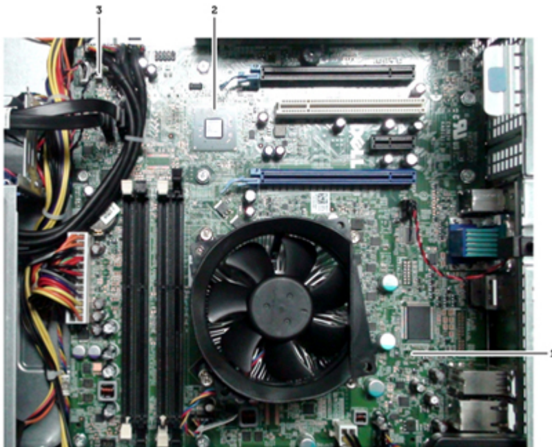
Obrázok 2. Systémová doska s odstráneným tepelným snímačom a chladičom
